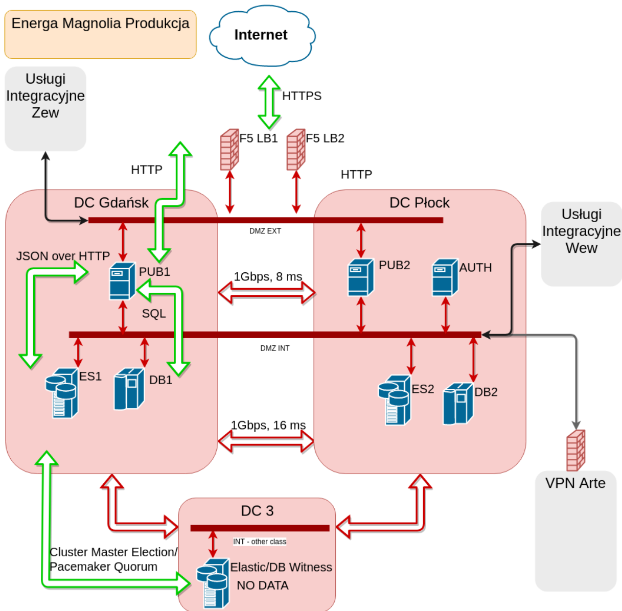
Rysunek Błąd! Nie określono sekwencji. - Architektura ogólna środowiska produkcyjnego
