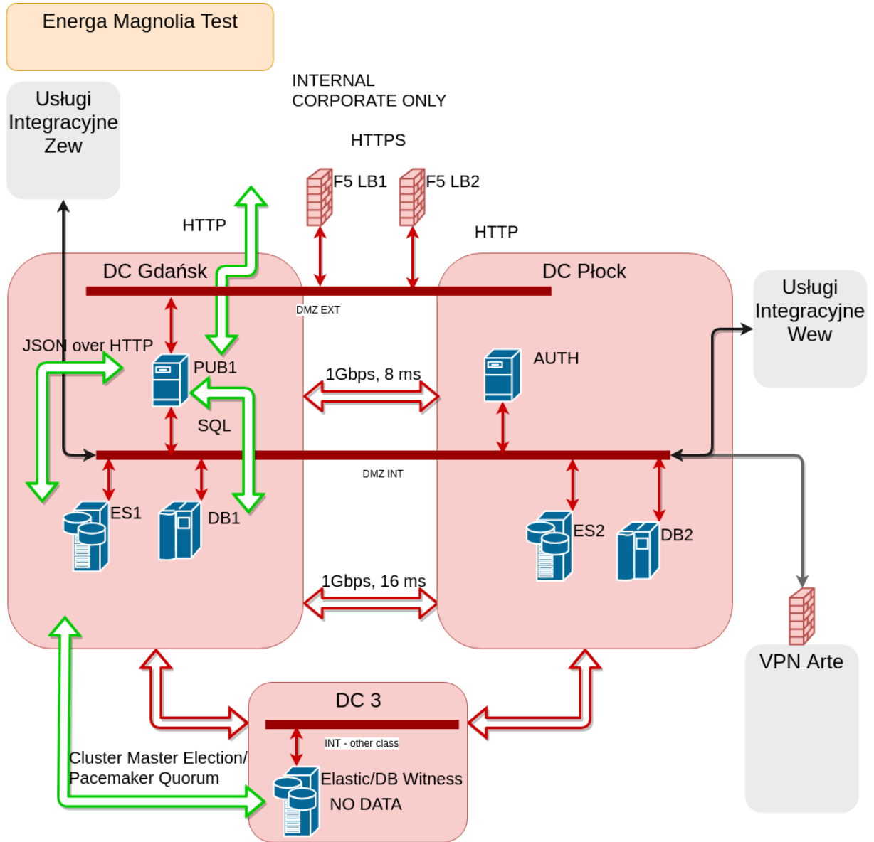
Rysunek Błąd! Nie określono sekwencji. - Architektura ogólna środowiska testowego
