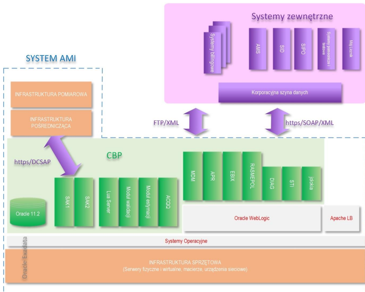
Rys 2) Poglądowy schemat architektury Systemu AMI oraz modułów aplikacji CBP (kolor zielony)
