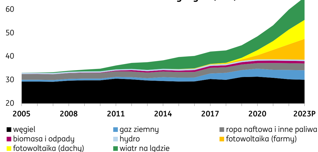
Moce zainstalowane w elektroenergetyce (GW)
