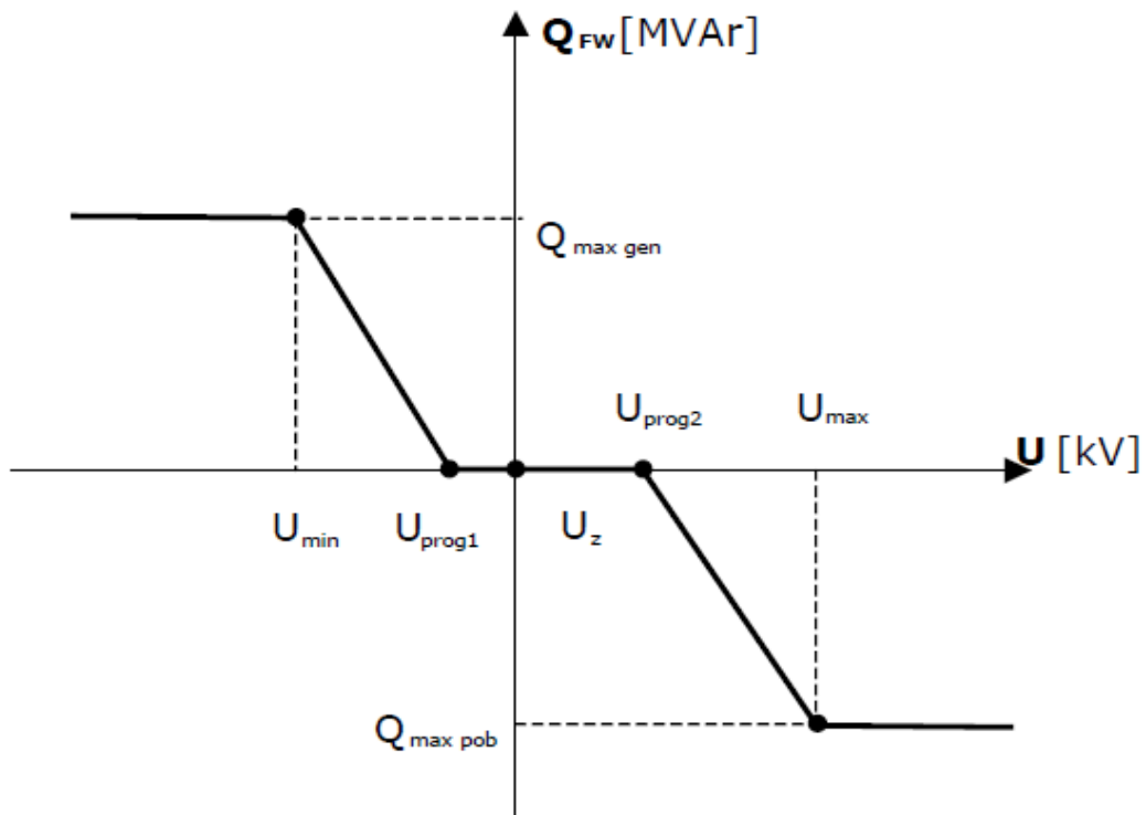
Rysunek 1 - Poglądowa charakterystyka statycznej regulacji
