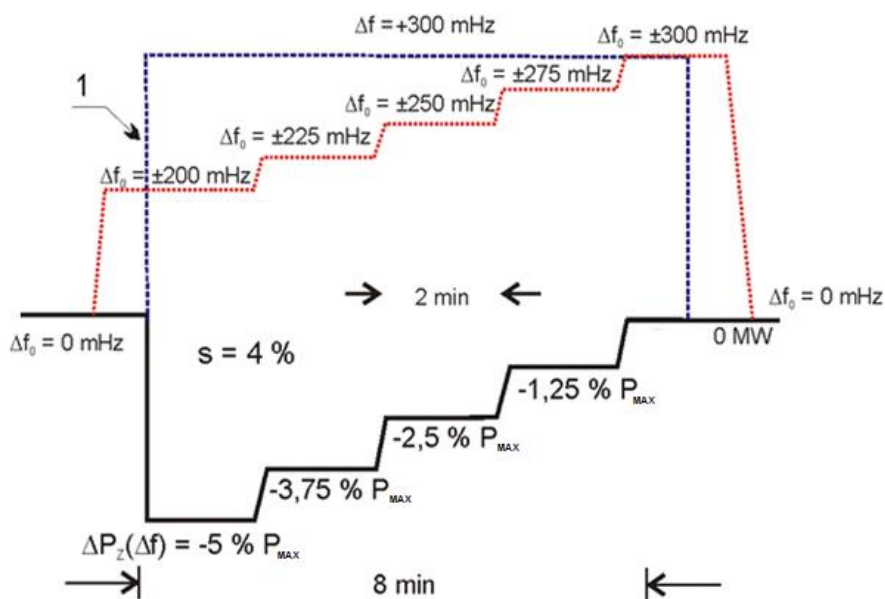
Rys. 4 Sprawdzenie odpowiedzi częstotliwościowej przy zmianach: strefy nieczułości odpowiedz częstotliwościowej, statyzmu oraz odchyłki częstotliwości
