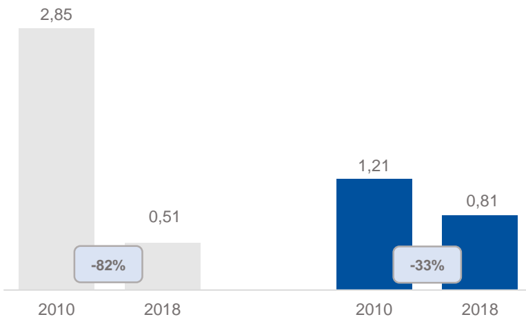
Emisyjność SO x [kg/MWh]
