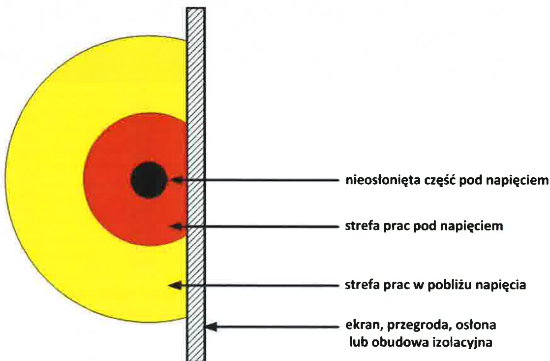
Rysunek Nr 2. Ograniczenie minimalnego odstępu w powietrzu poprzez zastosowanie sprzętu ochronnego
