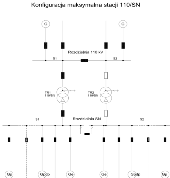
Rys.1. Konfiguracja maksymalna GPZ
