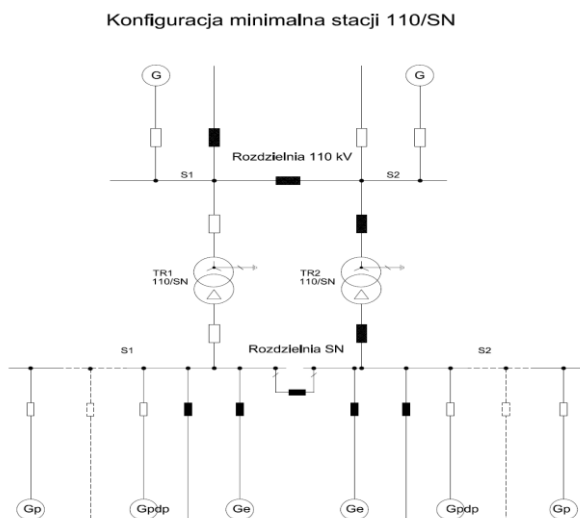
Rys.2. Konfiguracja minimalna GPZ
