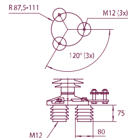
Podstawa izolacyjna
